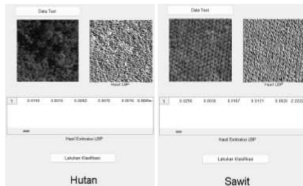
Gambar 4. Hasil Ekstraksi Fitur LBP
