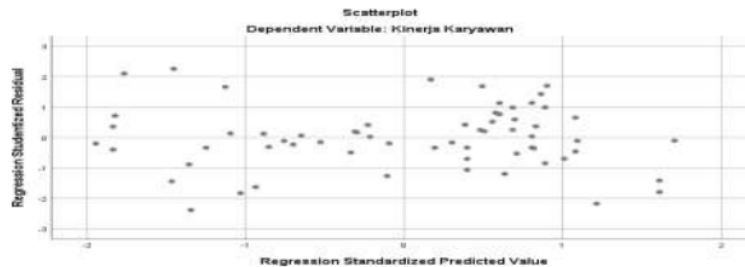
Gambar 2 Grafik Scatter Plot
