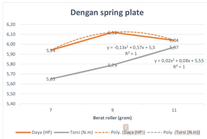
Gambar 4.2 Grafik Hubungan Daya (HP) dan Torsi (N.m) menggunakan Spring Plate Terhadap Berat roller
