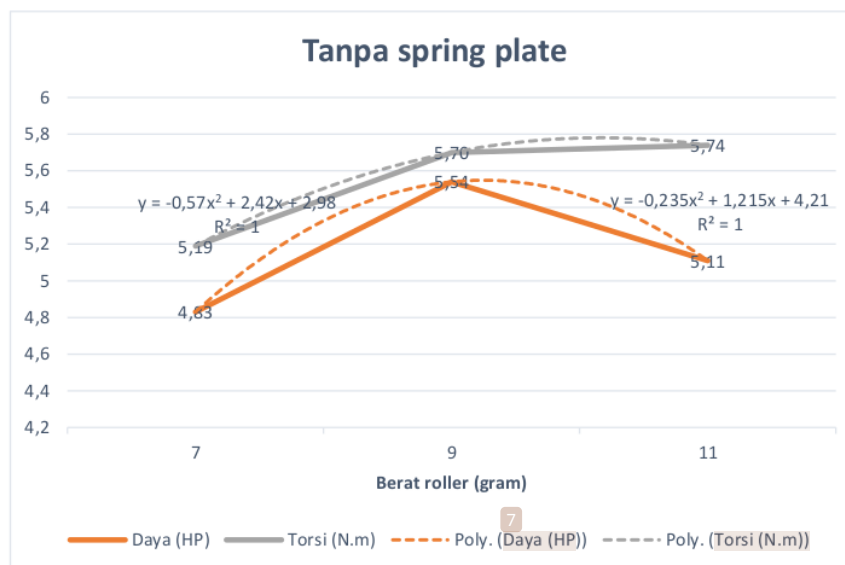
Gambar 4.1 Grafik Hubungan Daya (HP) dan Torsi (N.m) Tanpa Spring Plate Terhadap Berat Roller (gram)
