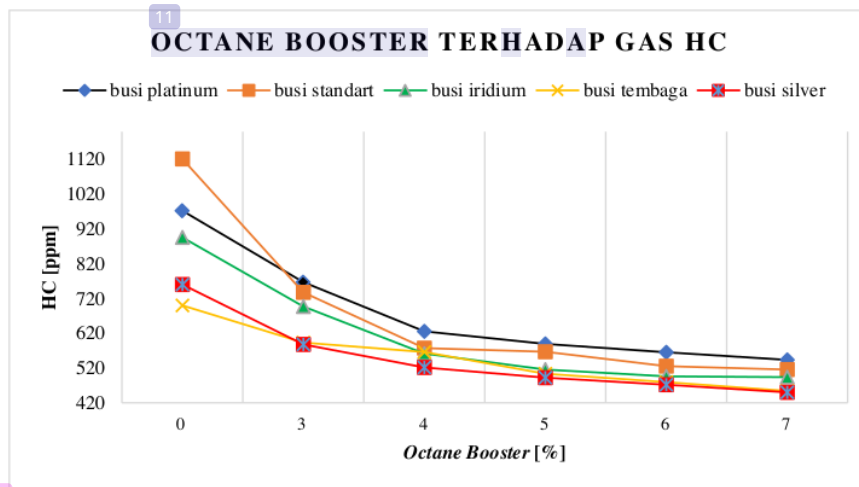
2 Gambar 2. Grafik Emisi Gas Buang HC pada Variasi Persentase Octane Booster
