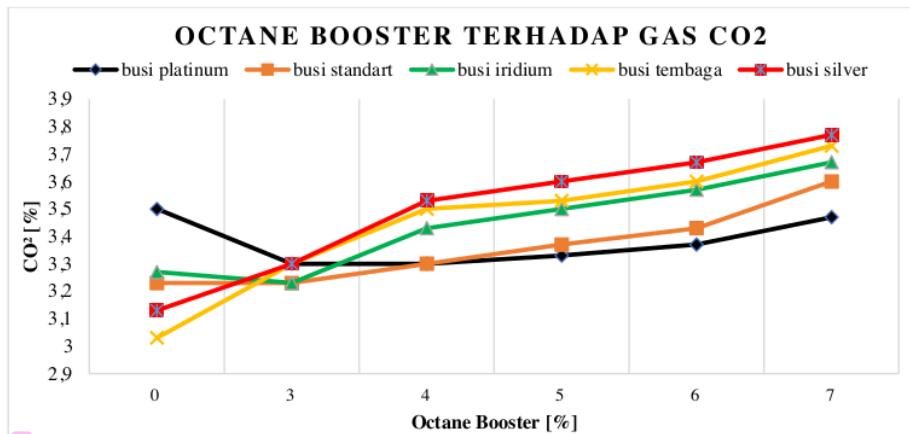
2 Gambar 3. Grafik Emisi Gas Buang CO 2 Pada Variasi Persentase Octane Booster
