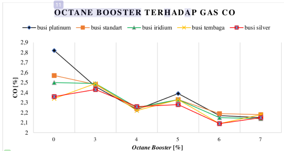
5 Gambar 1. Grafik Emisi Gas Buang CO pada Variasi Persentase Octane Booster
