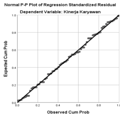
Gambar 1 Grafik Uji Normalitas P-Plot
