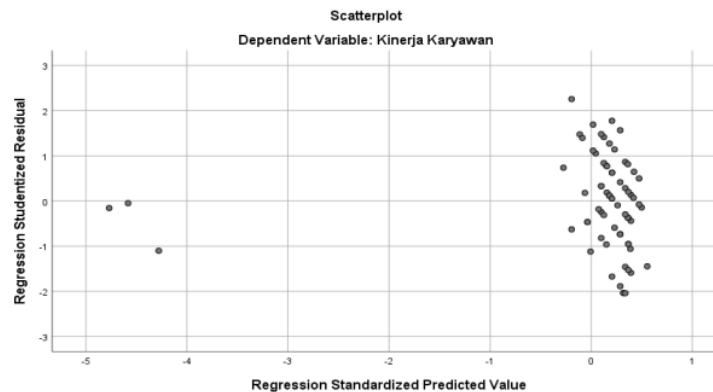
Gambar 2 Uji Heterokedastisitas Scatterplot
