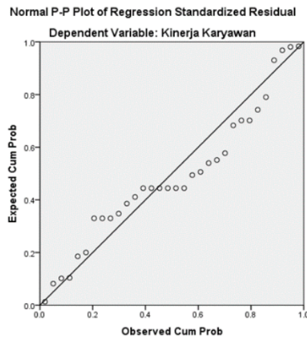
Gambar IV. 1 Hasil Uji Normalitas Grafik P-Plot
