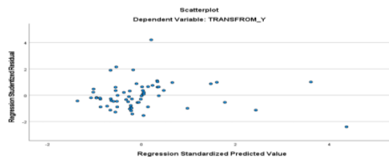
Gambar 1. Grafik Scatterplot
