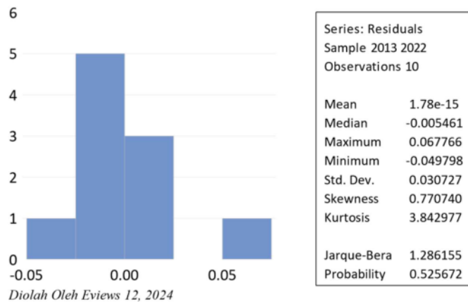
Gambar 1. Diagram Uji Normalitas
